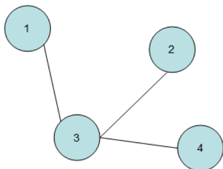
无向图
