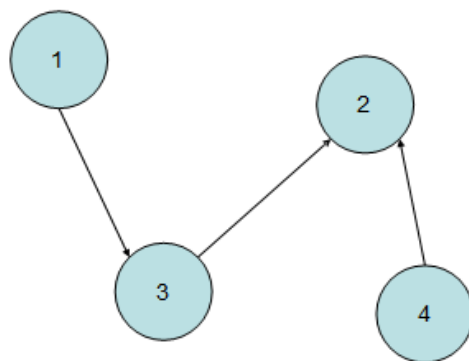
有向图
